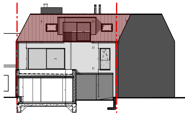
ACHTERGEVEL
